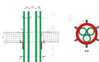
Rys. 8 Rekomendowana obudowa segmentowa
