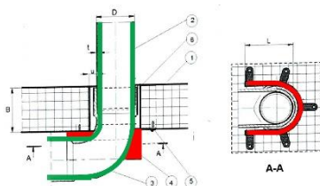
Rys. 7 Rekomendowana obudowa segmentowa
