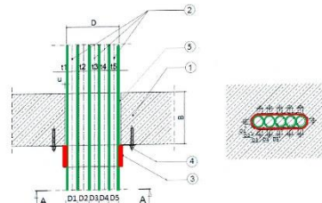
Rys. 9 Rekomendowana obudowa segmentowa
