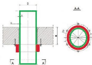
Rys. 4 Rekomendowana obudowa ciągła lub segmentowa
