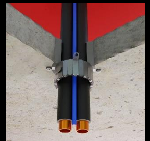
WIAZKI RUR METALOWYCH W IZOLACJI KACZUKOWEJ Z KABLEM
