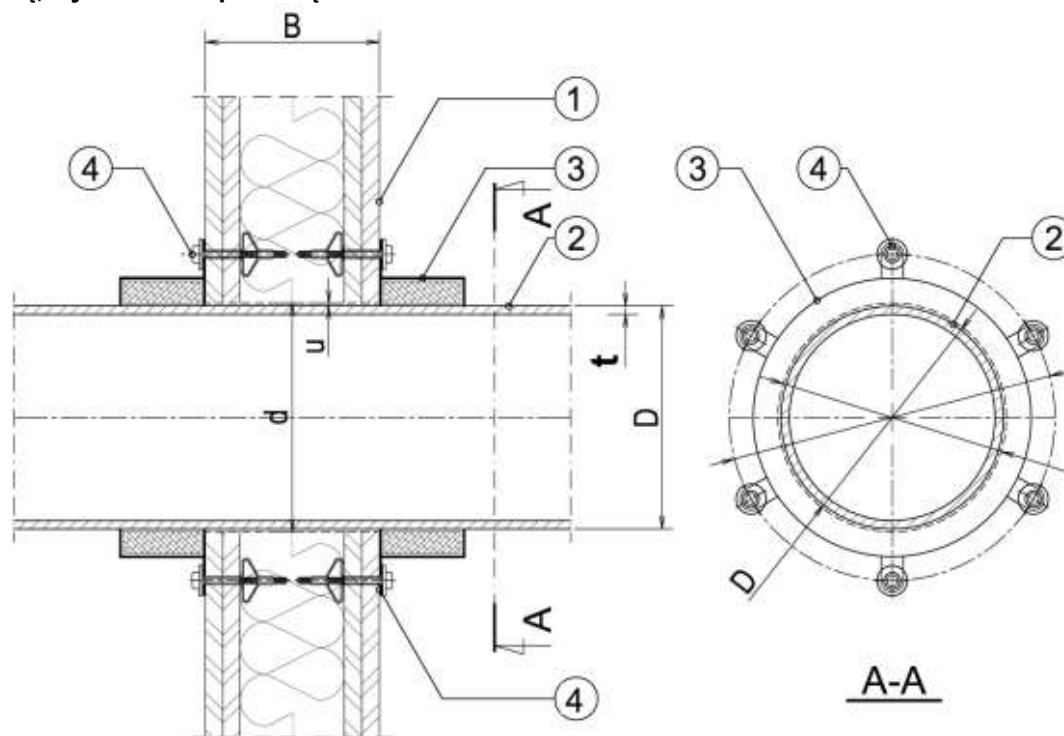
Rys. C3. Uszczelnienia przejścia instalacyjnego rury z tworzyw sztucznych przez ścianę podatną, wykonane za pomocą CarboCollar CC
