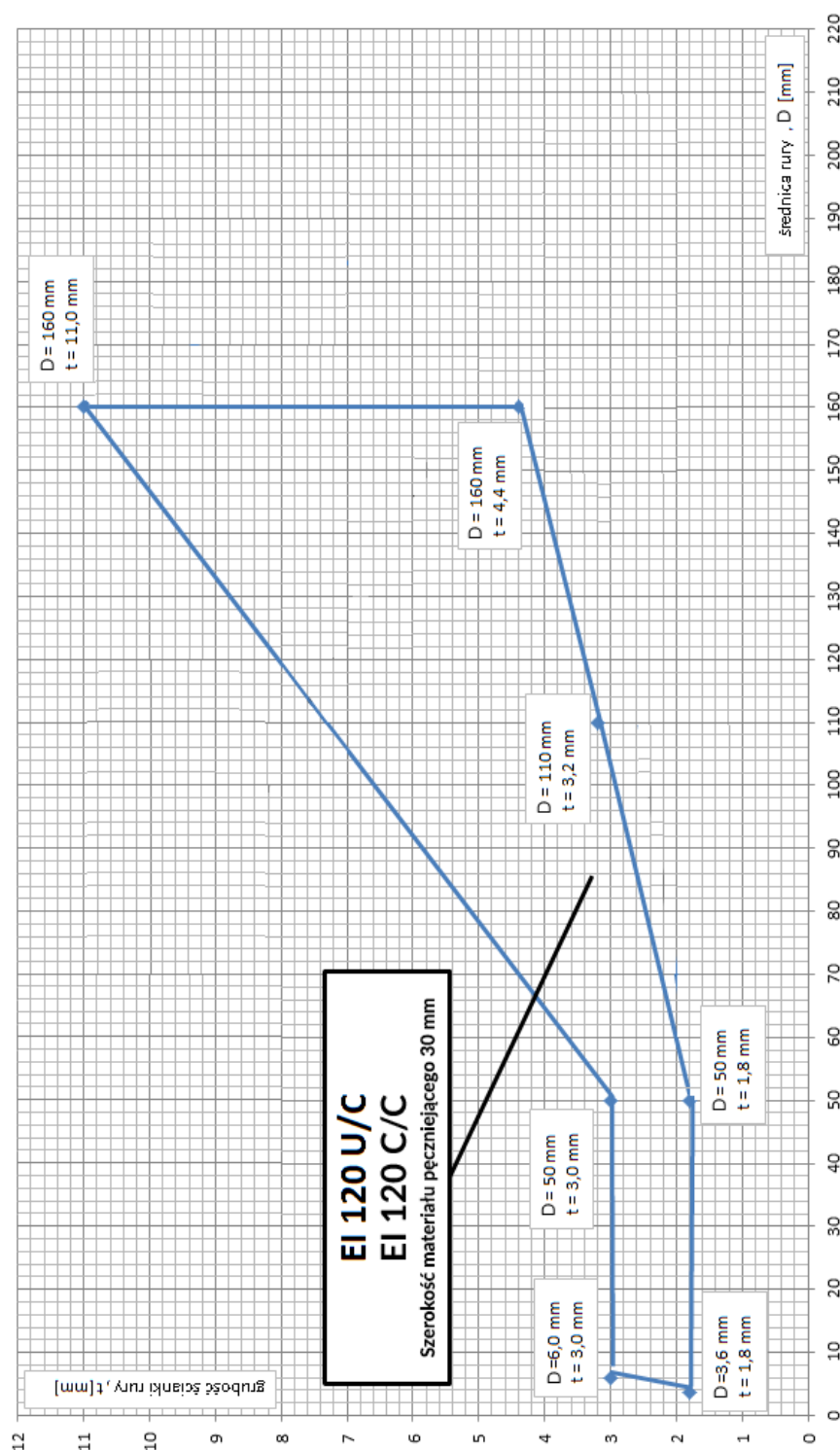
Rys. D58. Zakres przejść instalacyjnych rur z PVC-U/PVC-C uszczelnionych kołnierzami CarboCollar CC w ścianie sztywnej o grubości B \geq 125 mm, wykonanych wg rys. C2 w Załączniku C
