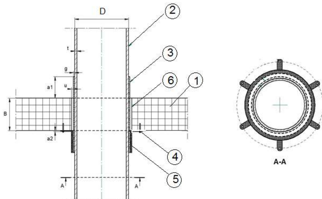
Rys. C20. Uszczelnienia przejścia instalacyjnego rur Wavin z izolacją PE przez strop sztywny, wykonane za pomocą CarboCollar CC
