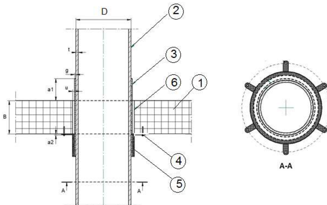
Rys. C8. Uszczelnienia przejścia instalacyjnego rur z tworzyw sztucznych z izolacją PE przez strop sztywny, wykonane za pomocą CarboCollar CC
