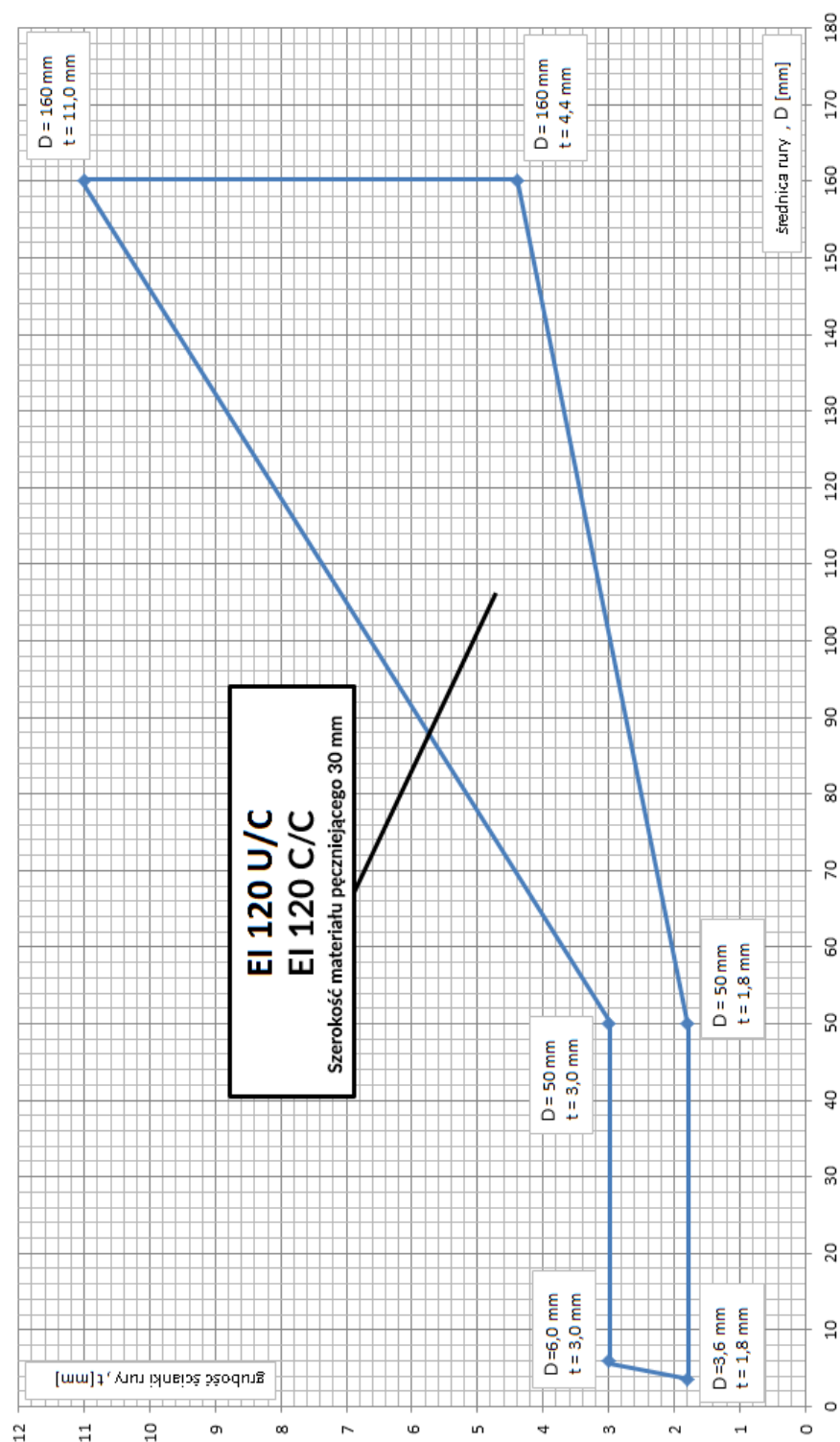
Rys. D57. Zakres przejść instalacyjnych rur z PVC-U/PVC-C uszczelnionych kołnierzami CarboCollar CC w ścianie sztywnej o grubości 100 \text{ mm} \leq B < 125 \text{ mm} , wykonanych wg rys. C2 w Załączniku C
