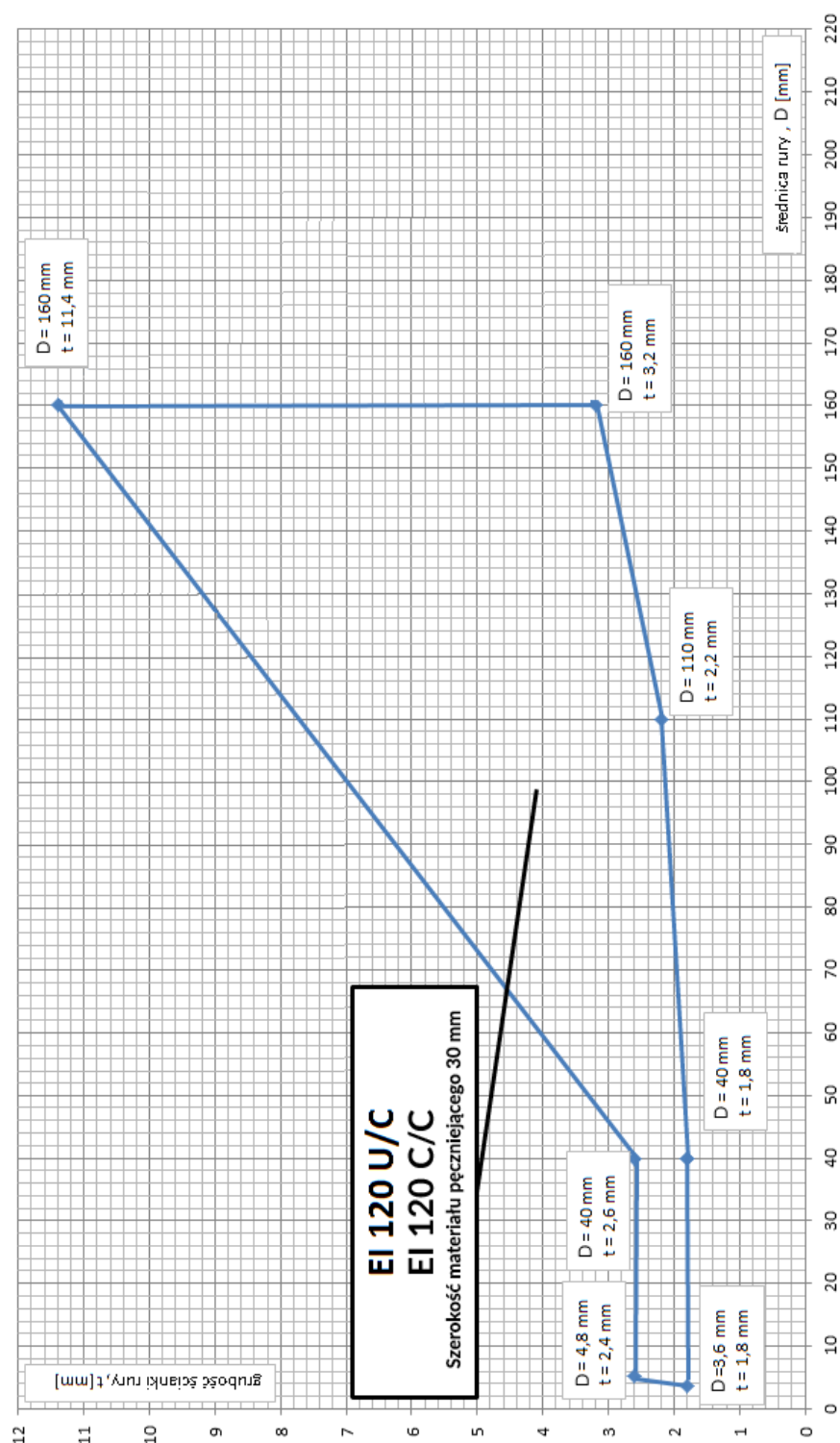
Rys. D55. Zakres przejść instalacyjnych rur z PP uszczelnionych kołnierzem CarboCollar CC w ścianie sztywnej o grubości B \geq 125 mm, wykonanych wg rys. C2 w Załączniku C
