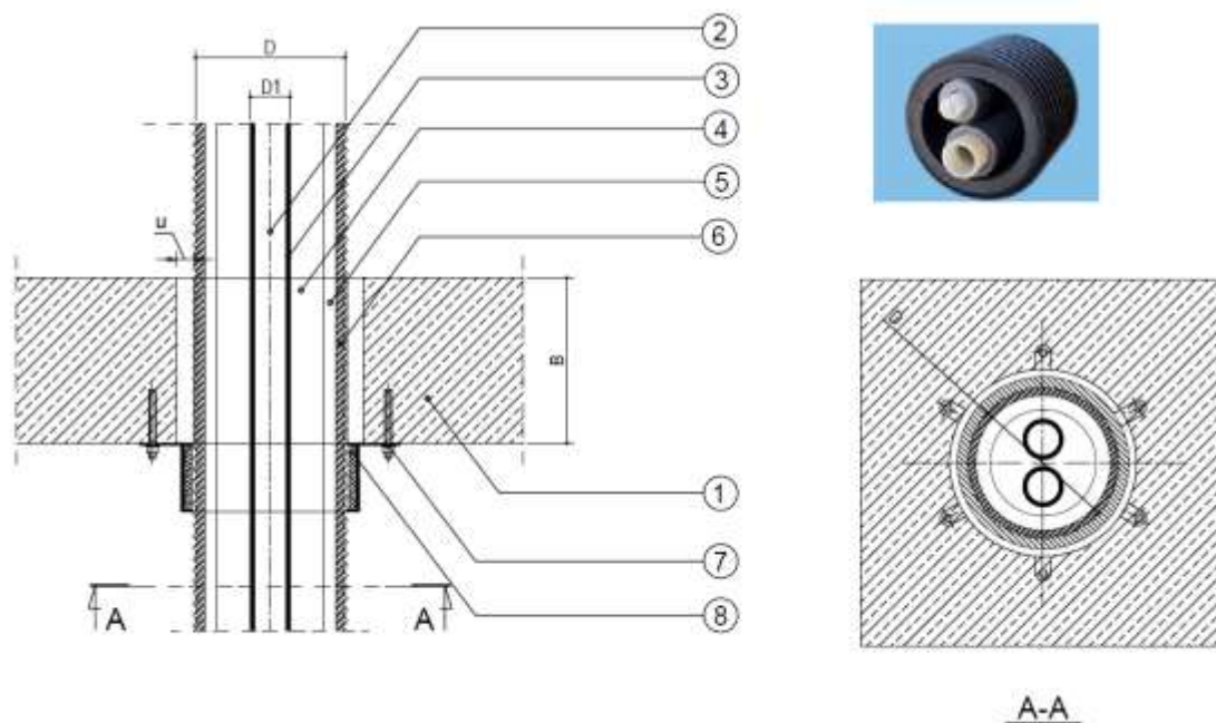
Rys. C13. Uszczelnienie przejścia instalacyjnego podwójnej rury grzewczej typu Syncopex C.O. PN6/95 C,C.W. PN10/70C z izolacją PE w stropie sztywnym, wykonane za pomocą CarboCollar CC
