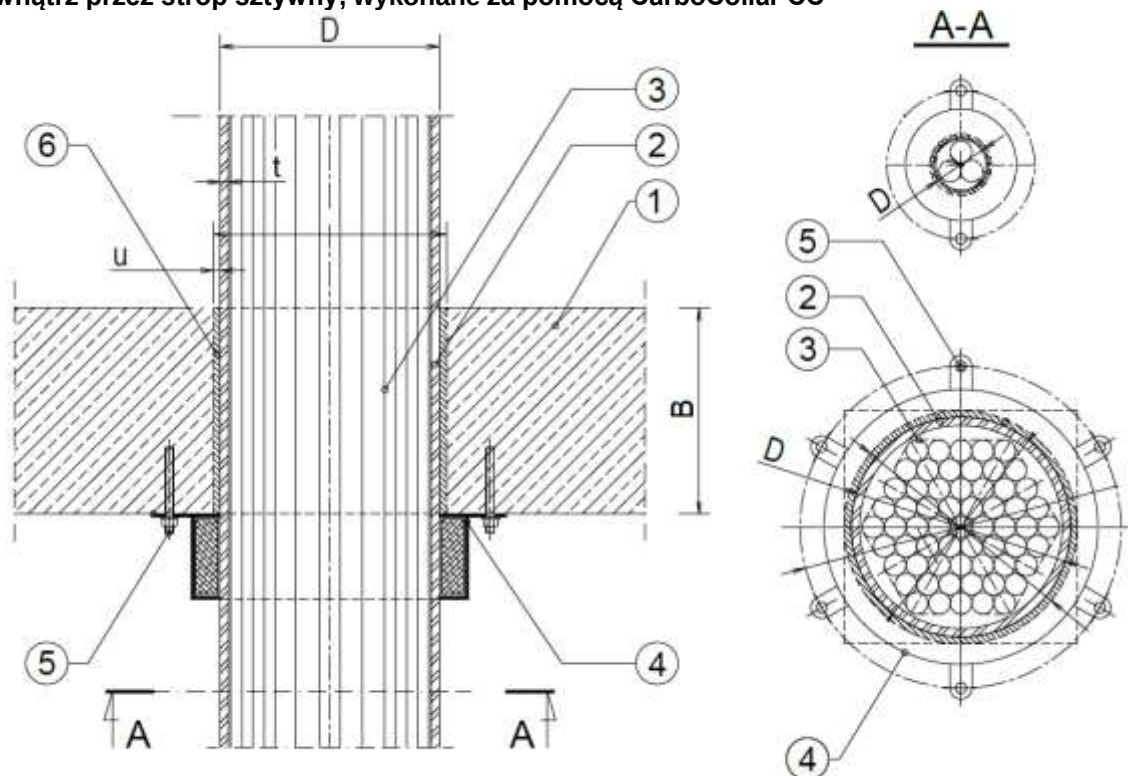
Rys. C7. Uszczelnienia przejścia instalacyjnego rur z tworzyw sztucznych z rurami z PP wewnątrz przez strop sztywny, wykonane za pomocą CarboCollar CC
