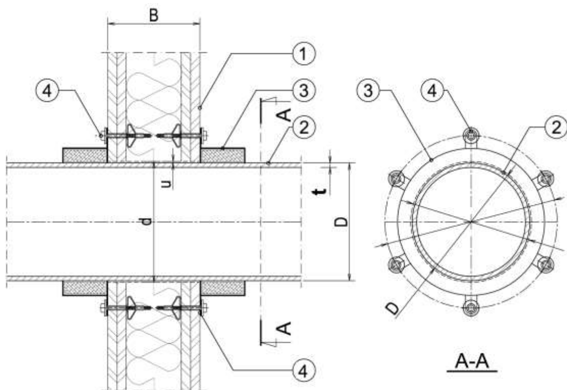
Rys. C17. Uszczelnienia przejścia instalacyjnego rur Wavin przez ścianę podatną, wykonane za pomocą CarboCollar CC
